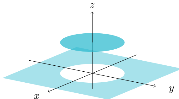
図 1.1 D = \{(x, y) \in \mathbb{R}^2 \mid x^2 + y^2 \leq 1\} \subset \mathbb{R}^2 の特性関数 \chi_D: \mathbb{R}^2 \rightarrow \{0, 1\} のグラフ
